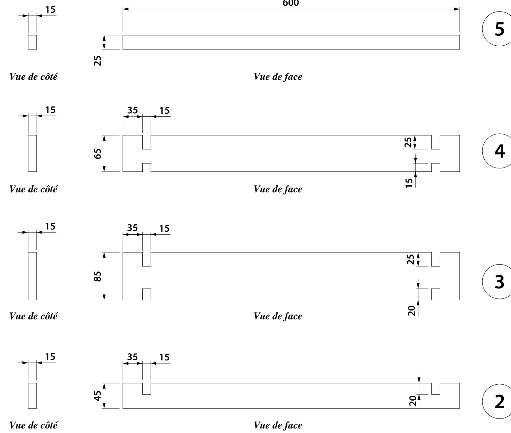
Lattes grand côté
