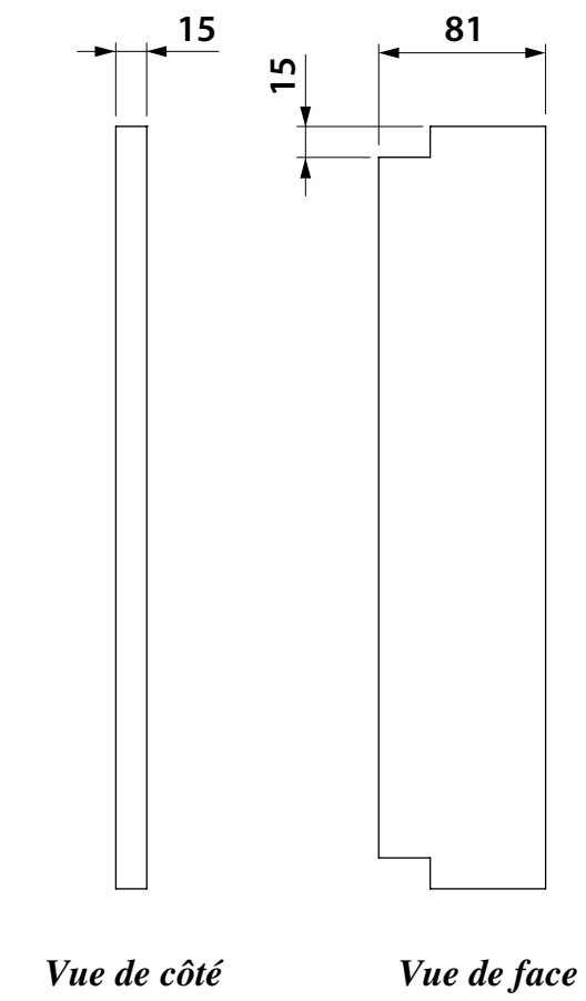
Latte de fond avec entailles
