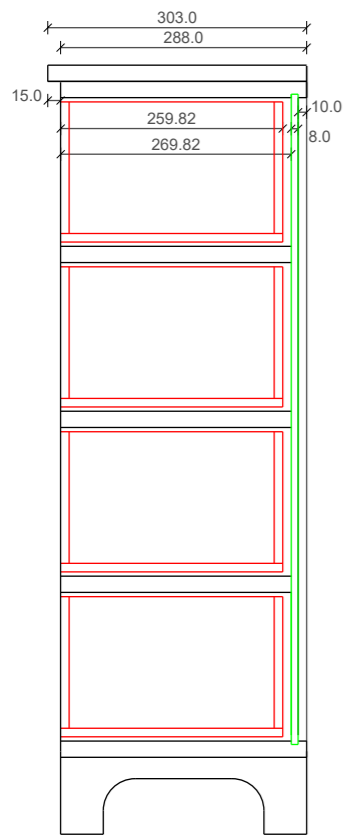
Coupe A-A
