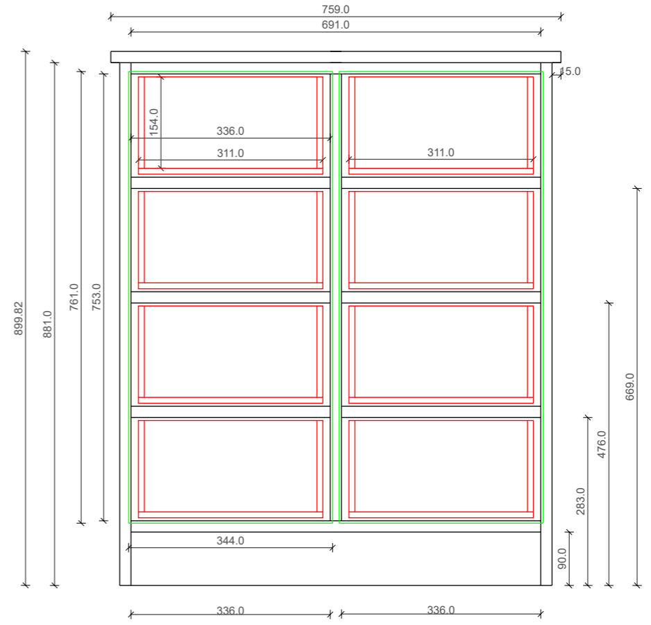
Coupe B-B
