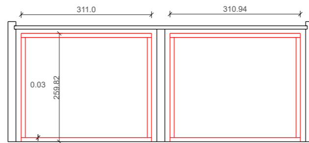
Coupe C-C
