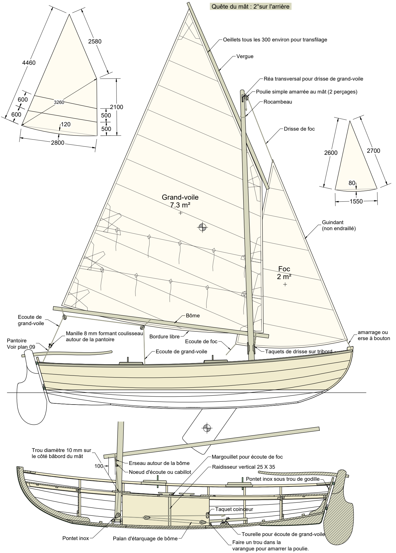
Mesker - Figure 12 Plan de voilure Echelle 1/30 et 1/80 François Vivier Architecte Naval
