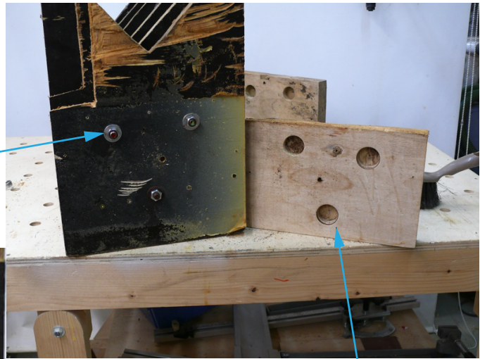
Plaque de protection des tiges filetées et des écrous. Perçage non débouchant permettant le passage des écrous.
